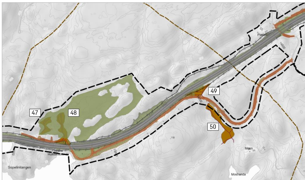
Figur 6-10: Oversikt over registrerte myrområder 47 til 50. Myrene ligger ved Vestre Hulldalsstranda og i Hulldalen. (Kilde: Sweco)
