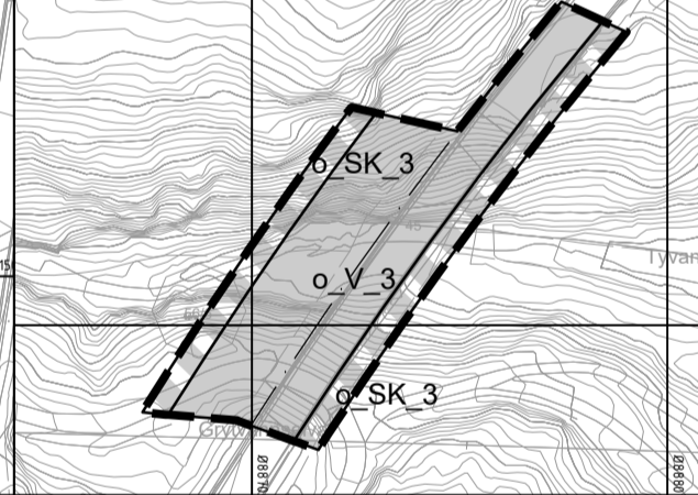
Vertikalnivå 3 - Iyvnanselva bru (1:2000)
