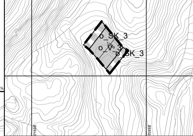
Vertikalnivå 3 - Hegland faunapassasje (bru/kulvert) (1:2000)
