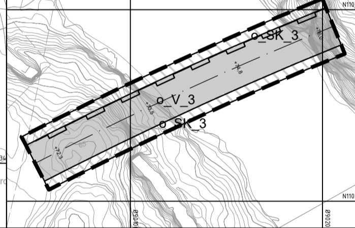
Vertikalnivå 3 - Tisjø bru (1:2000)
