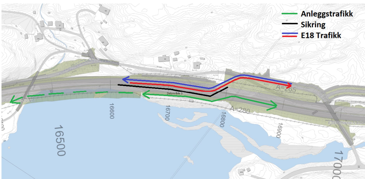
Figur 3-18: Midlertidig omkjøring E18 samt anleggstrafikk via rasteplass. (Kilde: Sweco).
