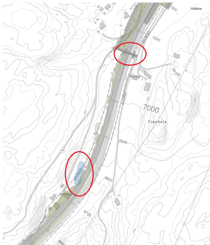
Figur 3-7: Fylling og arbeid i vann. (Kilde: Sweco).
