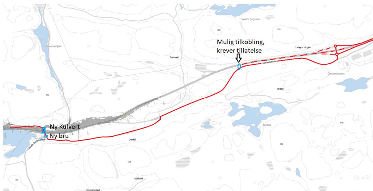
Figur 3-38: Midlertidig omkjøringsvei Gamla Sørlandske. (Kilde: Sweco).
