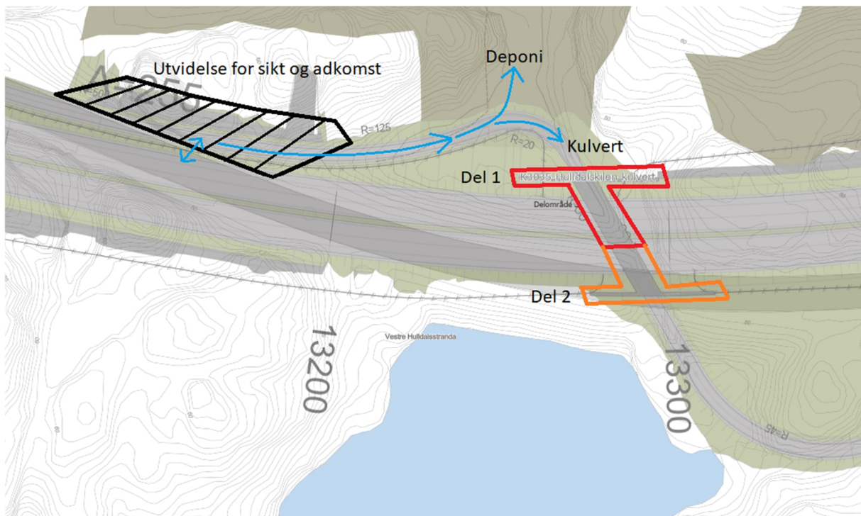
Figur 3-25: Anleggstekniske tiltak for bygging av Huldalskilen kulvert. (Kilde: Sweco).
