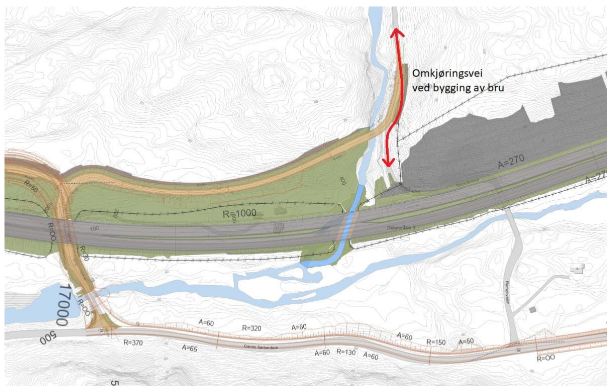
Figur 3-41: Midlertidig omkjøring ved bygging av bru. (Kilde: Sweco).
