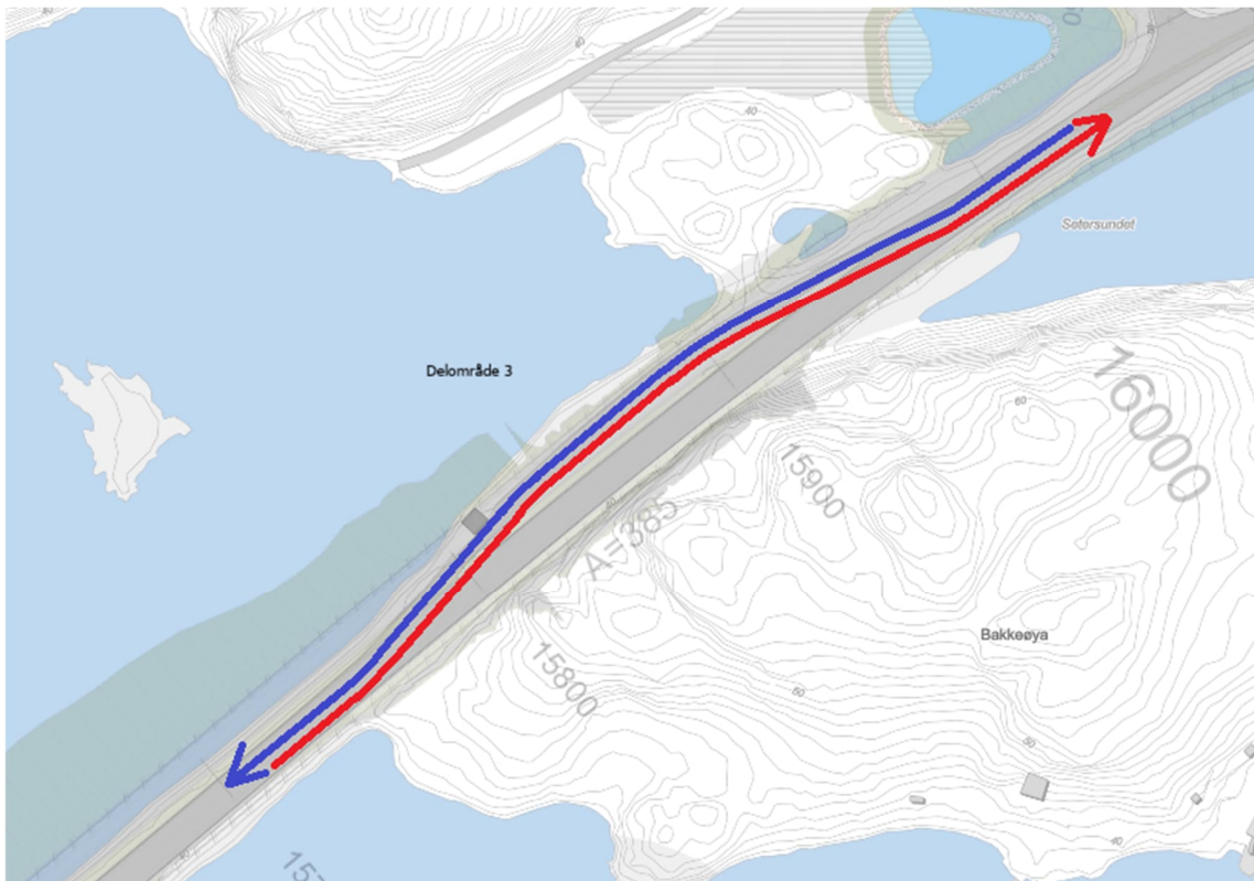
Figur 3-17: Midlertidig omkjøring via rasteplass under sprengning i Bakkeøya. (Kilde: Sweco).
