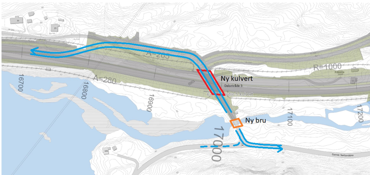
Figur 3-40: Midlertidig omkjøringsvei via Gamle Sørlandske og ny kulvert. (Kilde: Sweco).
