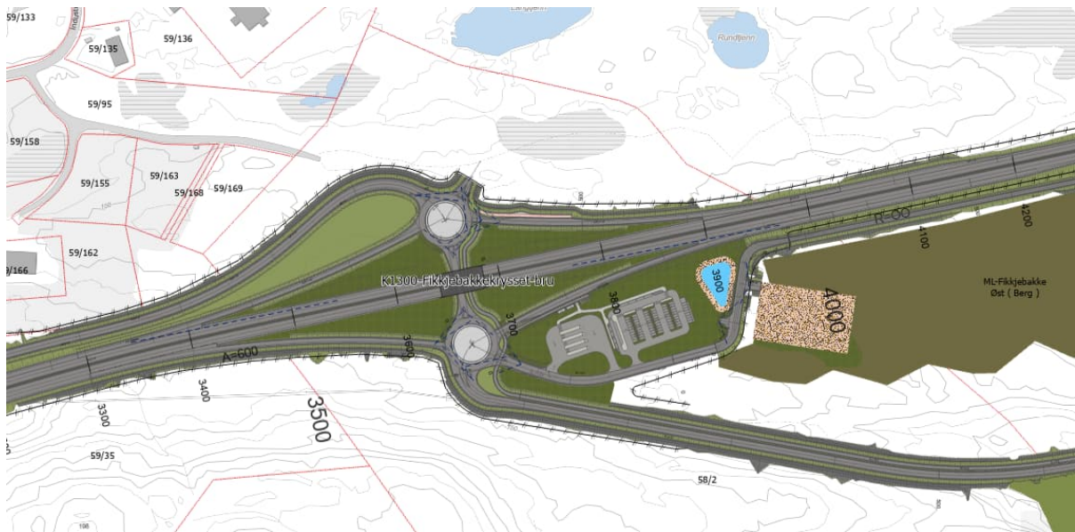
Figur 3-8: Kryss Fikkjebakke. (Kilde: Sweco).
