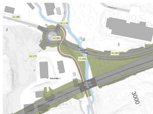
Figur 3-7: Rundkjøring Fikkjebakke på eks. Krokenveien ved adkomst til industriområdet. (Kilde: Sweco).
