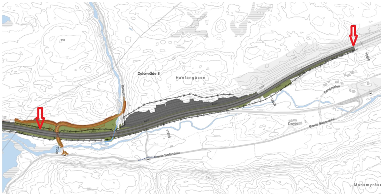
Figur 3-37: Delstrekning 6, Gongelva – Dørdall. (Kilde: Sweco).
