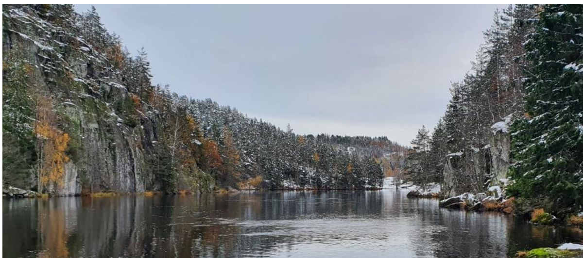
Figur 4-12 Tisjø bru – brustedet sett mot sør. På østsiden, dvs. til venstre i bildet, er berget svært bratt. Brua vil krysse over omtrent midt i bildet i ca. 36 m høyde. Normalvannstand i Tisjø er på kote +37,3. (kilde: Sweco)
