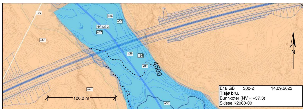
Figur 4-13 Tisjø bru – bunnkotekart (anleggsvei og midlertidige fyllinger ikke vist).
