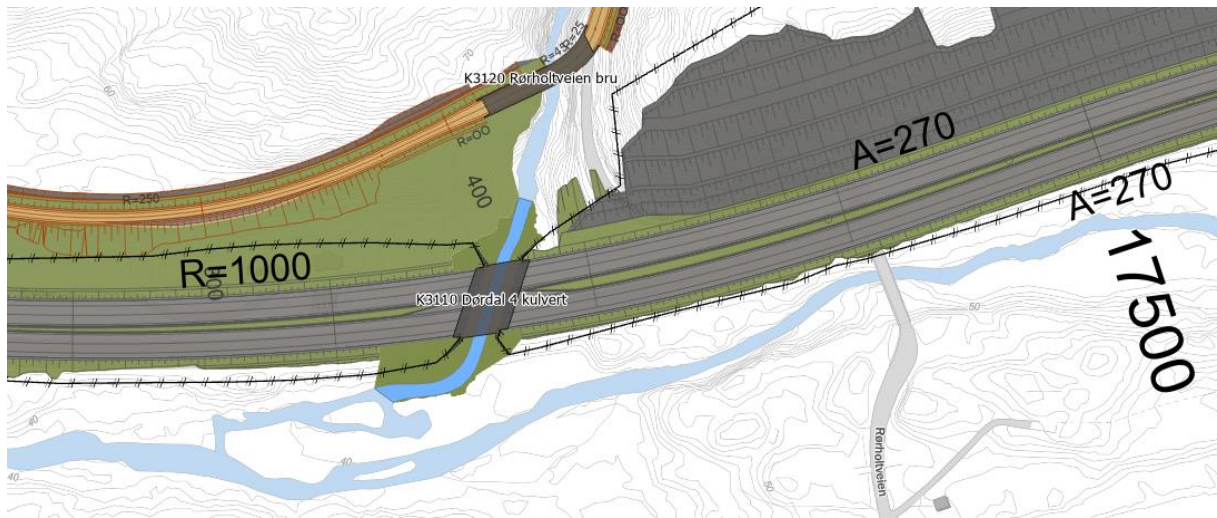
Figur 4-27 Dørdal 4 kulvert – faunapassasje under E18. Grasdaltjennbekken kommer ned fra nord og munner ut i Gongelva som renner vestover mot Bakkevann langs sørsiden av E18.
